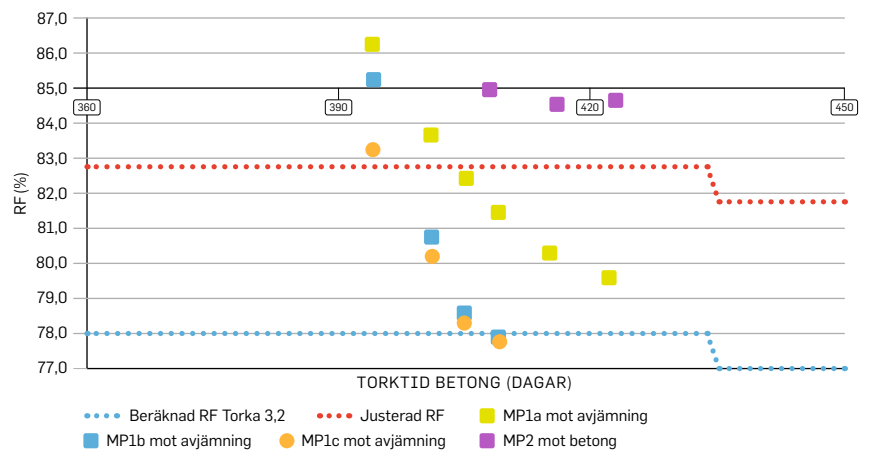
FIGUR 3 Trippelpunkt monterad mot torr avjämnning visar helt annan uttorkningshastighet än mätpunkt 2 där avjämnningen bilats bort.
