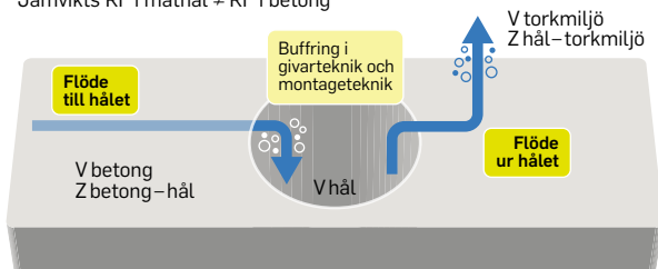
FIGUR 2 Principer för jämvikt i ett mäthål. Ånghaltsskillnaden (Vbetong-Vhåll) måste vara nära noll för att kunna mäta hur blöt betongen är via fuktmätning i hålet.
