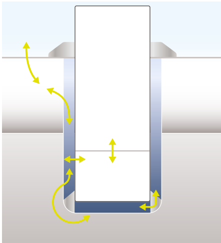
FIGUR 2 Läckagevägar runt borrhålstätningar går i alla riktningar. Mängden betong som bromsar läckaget kan bli kraftigt reducerat vid ängöppna pågjutningar där fukten lätt transporterar sig förbi övre tätningen.
