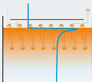
Figur 5. Ventilera system hanterar både fukt och emissioner bra. Då golvet är helt separerat från underlaget är alkali normalt inget problem heller.
