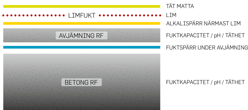
Figur 10. Placering av spärrar i limmat golv. En alkalispärr fungerar bara bra om det inte ligger alkaliskt material ovanför den. En ångspärr måste ha en fuktbuffert ovanför sig för att kunna hantera limfukt bra.
