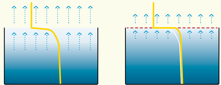
Figur 3. Fuktprofiler beroende på ytbeläggningens täthet. I en konstruktion som torkar mot en torkmiljö är det blötest nere i konstruktionen medan fukt lämnar ytan. En fuktprofil (gul linje) bildas
