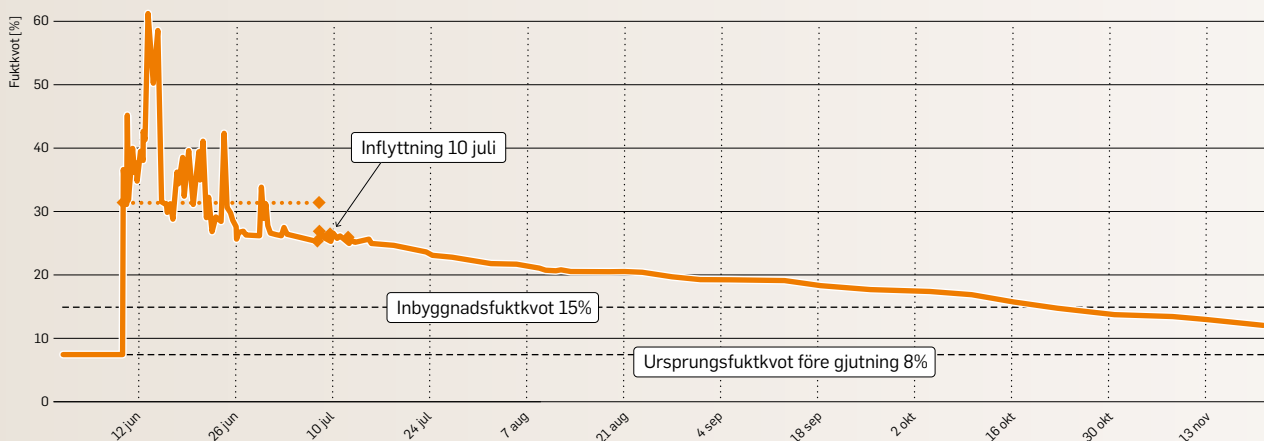
Figur 14. Fuktkvot (Obs. indikativ mätning då densiteten för spånskiva ≠ furuträ) i spånskiva som begjuts med 30mm självttorkande avjämningsmassa och tätskikt efter 24 h.
