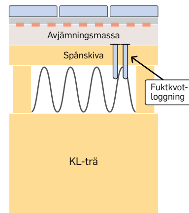
Figur 13. Sektionsskiss som illustrerar fuktkvotsloggningen i projekt.
