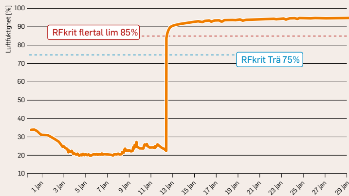
Figur 9. Mätresultat i jämförelse med några vanliga fuktgränsvärden.
